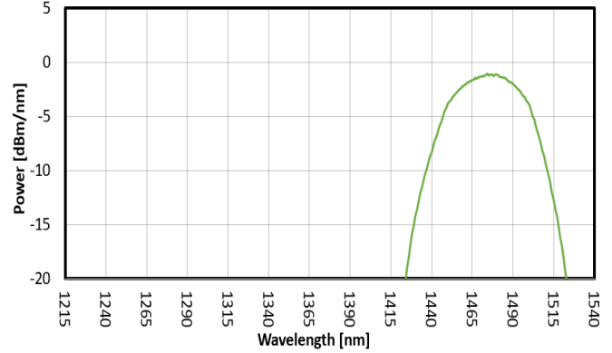
FIG. 2: SLED 1 SPECTRUM
